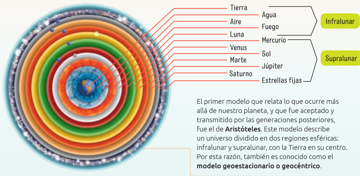
➡ Modelo planetario de Aristóteles. La representación no está a escala.
