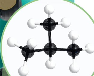
2-metilpropano
